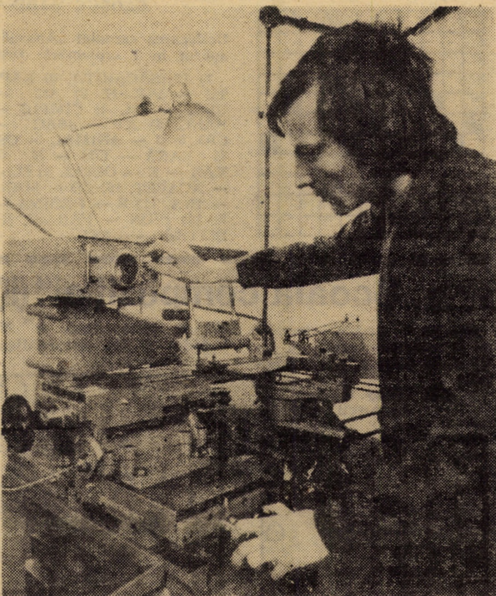
La o mașină de rectificat profile din atelierul scularie al întreprinderii „Flamura roșie” Sibiu, utecistul Dumitru Moțoc realizează S.D.V.-uri cu un înalt grad de precizie, numărîndu-se printre tinerii cu o bună pregătire profesională, fapt care i-a permis să urmeze cursurile serale de subingineri ale Facultății de mecanică Sibiu
