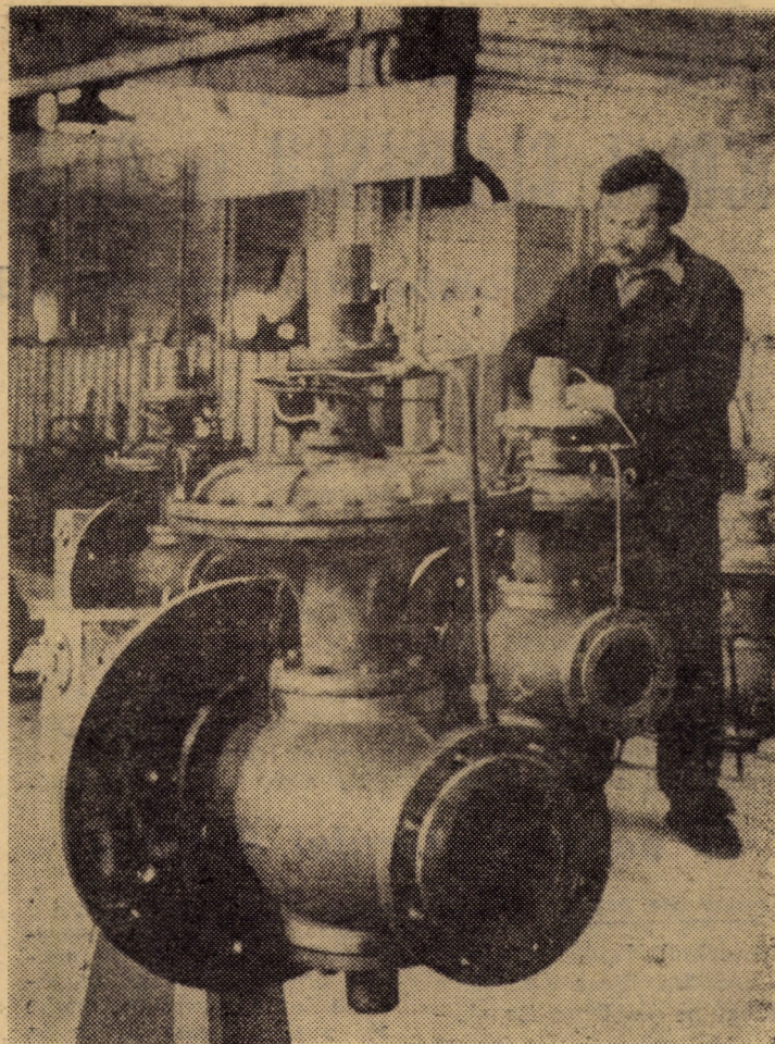
Imagine de la Uzina mecanică gaz metan Mediaș Foto: H. BUCHFELNER
