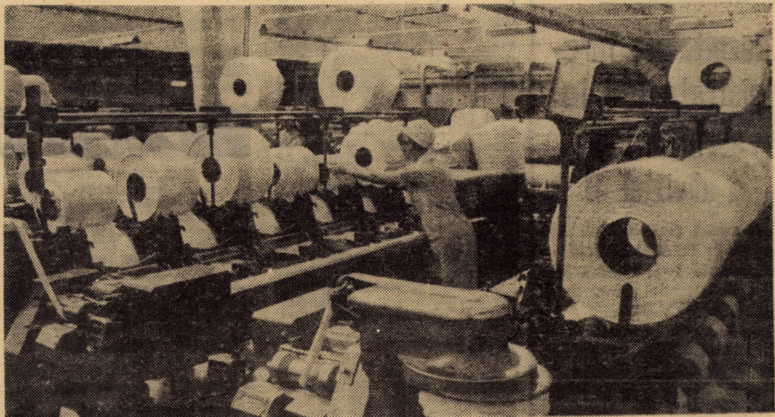
Secția filatură a întreprinderii „Firul roșu” Tâlmăciu. Grupul de mașini de pieptănat, unde sînt eliminate fibrele scurte din banda de bumbac Foto FR. NUSS
