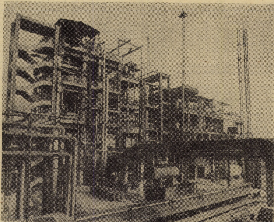
Carbosin Copșa Mică - Instalația de sinteză a metacrilatului de metil
