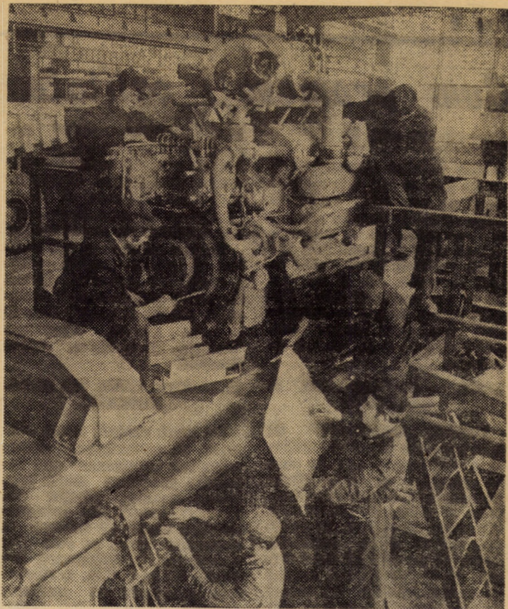
Montarea motorului pe infrastructură la autobasculanta de 100 tone. Lucrarea o efectuează echipa condusă de maestrul Emil Szanto din secția montaj general a Întreprinderii mecanice Mirșa
