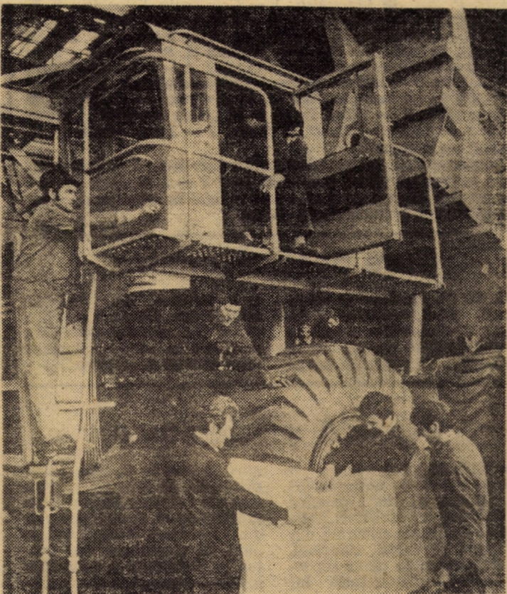
Înainte expedierii la beneficiar — echipe speciale verifică minuțios elementele de comandă hidraulică sau alte sisteme la bascula de 50 tone. În fotografie membrii echipei de finalizare din secția montaj general a Întreprinderii mecanice Mirșa Foto: FRED NUSS
