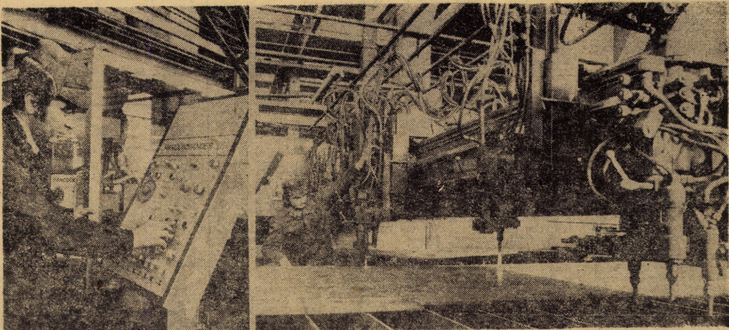
Harnicul colectiv de muncă al atelierului subansamble de la întreprinderea mecanică Mirsa se confruntă azi cu utilaje de tehnică avansată și de mare randament cum este mașina de debitat oxigaz automată, prin coordonate. În foto: sudorul specialist Aurel Căpătină (stînga) la pupitrul de comandă al instalației și sudorul Andrei Lalinca, regînd flacăra oxigaz. Foto: FRED NUSS
