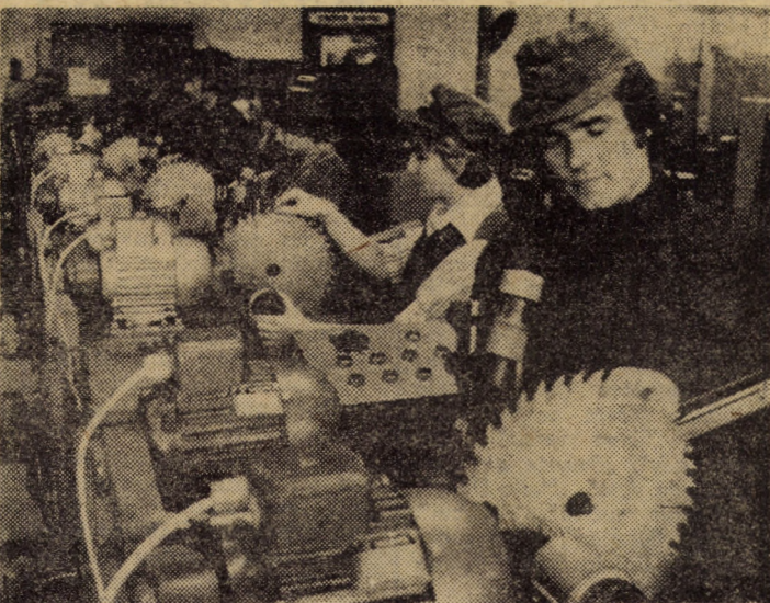
Noua linie de mașini de ascuțit fețe laterale la plăcuțele din carburi metalice, realizate prin autodotare de către un colectiv de specialiști din cadrul întreprinderii I.U.P.S. Sibiu
