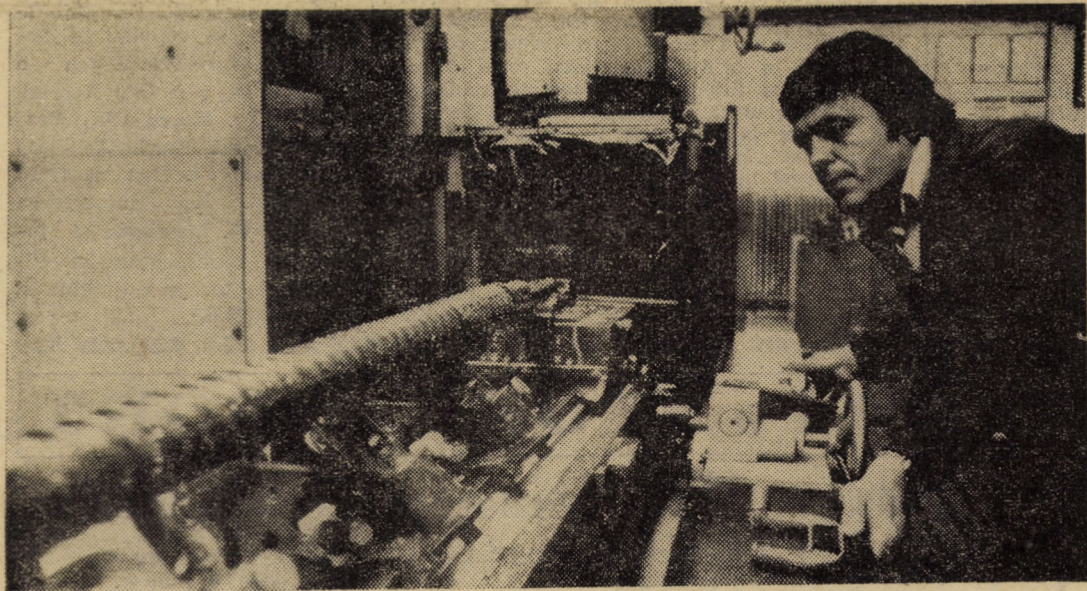
Lucrînd la unul din cele mai complexe utilaje din secția sculărie de la I.P.A. Sibiu — mașina de rectificat caneluri — comunistul Octavian Micu se remarcă la locul său de muncă prin conștiințozitate, perseverență și o bună pregătire profesională. Foto: FRED NUSS
