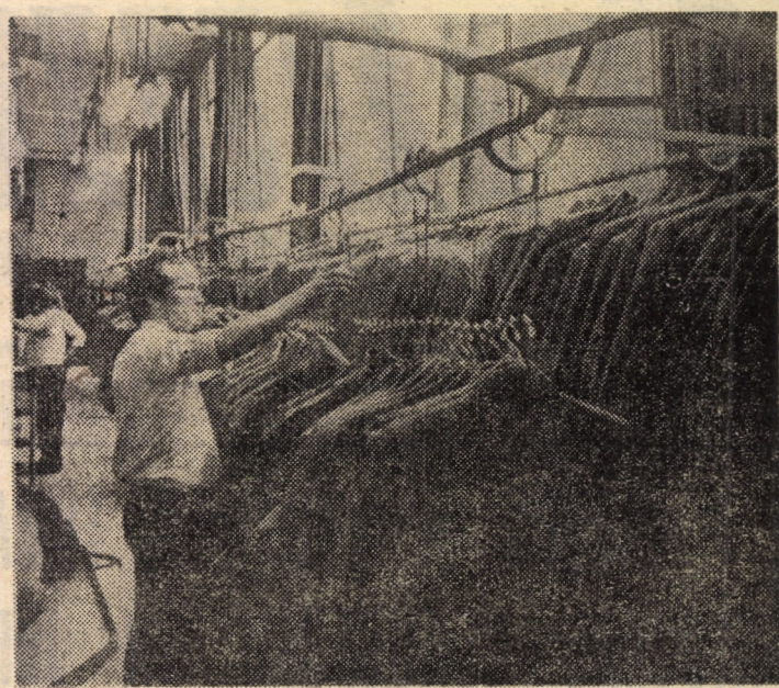
În vederea reducerii gradului de șifonabilitate a produselor, precum și a efortului fizic, în atelierul finisaj al întreprinderii de confecții „Steaua roșie“ Sibiu a fost realizată recent o linie de transport suspendată în zona de finisare a sacourilor
