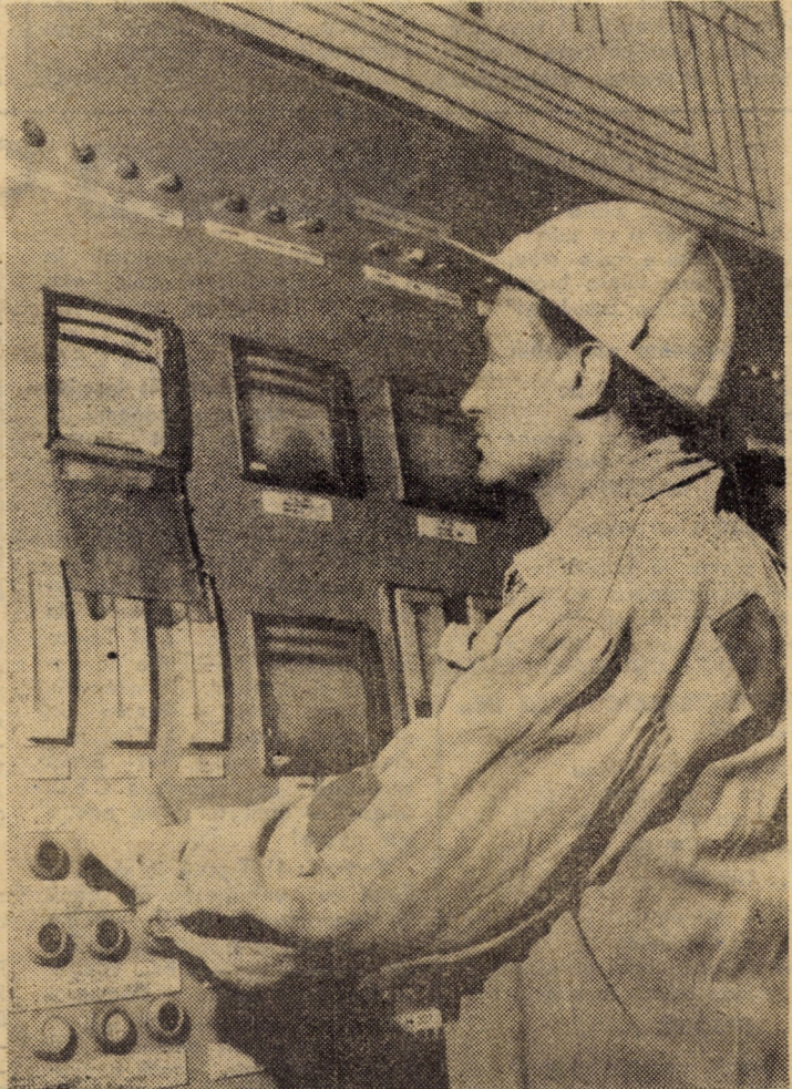
Supravegherea parametrilor în camera de comandă a furnalului la I.M.M.N. Copsa Mică. Foto: FRED NUSS
