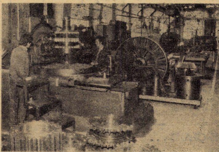
Vedere parțială a halei strungărie a întreprinderii „Independența” Sibiu. Foto: FRED NUSS
