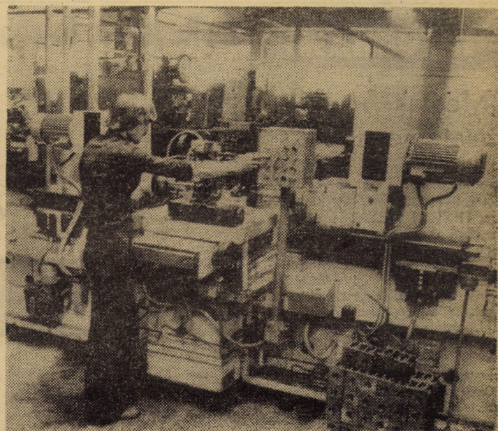
Agregatul de prelucrat alezaje capăt la corpurile distribuitoare — utilaj modern, automatizat, realizat în țară, instalat de curînd într-unul din atelierele de producție ale Fabricii de elemente hidropneumatice Sibiu Foto: Fred NUSS
