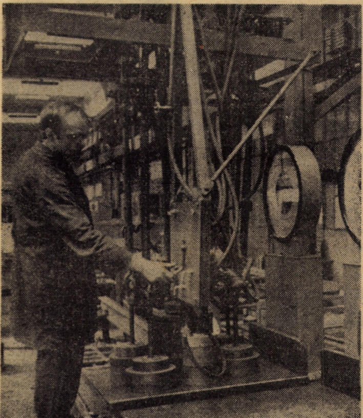
Înainte de a fi livrate beneficiarilor, basculele semiautomate sînt verificate și etalonate cu precizie. Întreprinderea „Balanta” Sibiu dispune în acest scop de standuri de încercări și aparatură complexă de verificare. În imagine: standul de etalonare a basculelor semiautomate Foto: Fred NUSS
