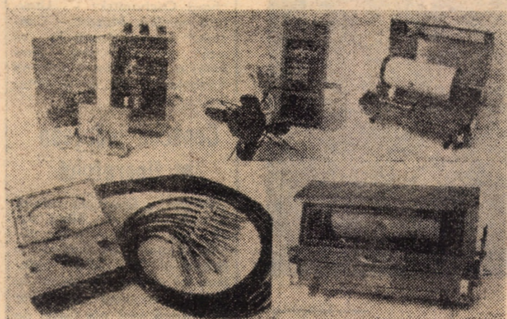
Aporatură hidro-meteorologică realizată de către colectivul Sibiu al Institutului de meteorologie-hidrologie. Higrometrele, pluviometrele, termometrele electronice de sol și alte asemenea aparate realizate la Sibiu înlocuiesc costisitoare importuri
