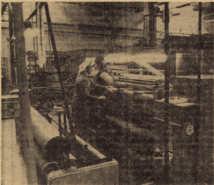
Întreprinderea textilă „Dumbrava” Sibiu. La o mașină de țesut mochetă netedă, tip „SCHUSSPOL”, utilaj de mare productivitate, țesătorele Raveca Bucur și Maria Cimpean realizează mochetă din fire mulate — un nou produs, recent apărut pe piață
