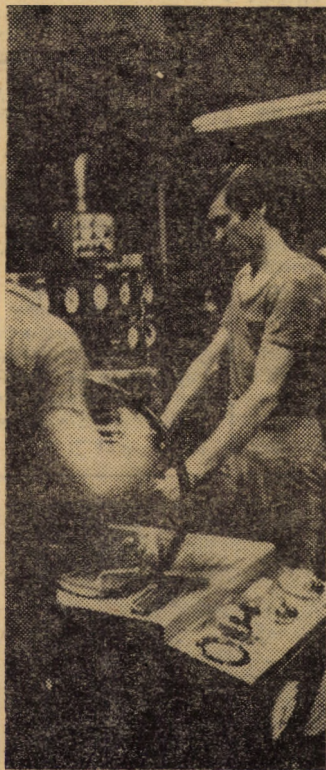
I.P.A. Sibiu. În imagine — stand de probă pentru componente destinate autocamioanelor
