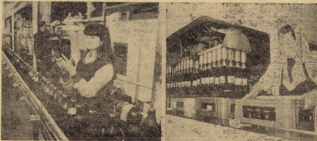
La întreprinderea de bere și amidon Sibiu a fost pusă în funcțiune recent o linie de pasteurizat în flux continuu de tip CONTIPA-12 cu o capacitate orară de 12 000 sticle bere. În imagine: linia de imbuteliere și de pasteurizare a berii
