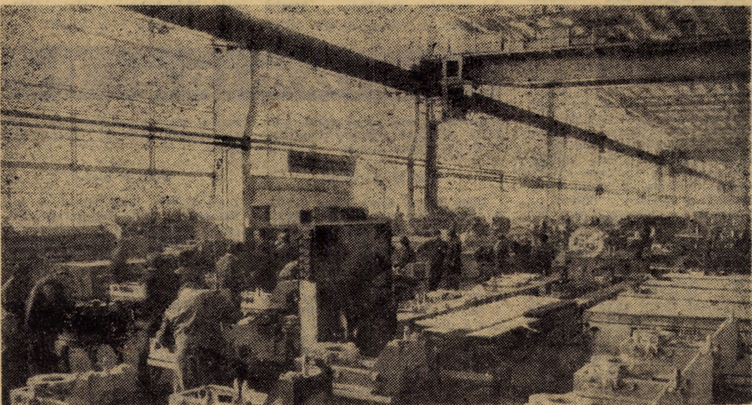
Prin munca de zi cu zi, harnicul colectiv de muncitori ai fabricii de utilaj metalurgic și turnătorii Sibiu întîmpină marile evenimente politice ale acestui an cu aoi și noi succese. În fotografie: aspect din hala de montaj
