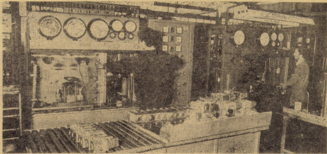
Întreprinderea de elemente hidro-pneumatice Sibiu. Unul din standurile de probă pentru distribuitoarele hidraulice la care se verifică pierderile de debit și presiune, funcționarea electromagnetelor, etc.
