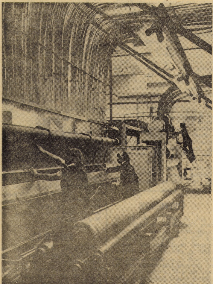
Întreprinderea textilă „Dumbrava”, Sibiu: mașini de țesut covoare „Tufted”. Aici se realizează produse de înaltă calitate, ce întrunesc cele mai exigente pretenții ale beneficiarilor Foto: Fred NUSS
