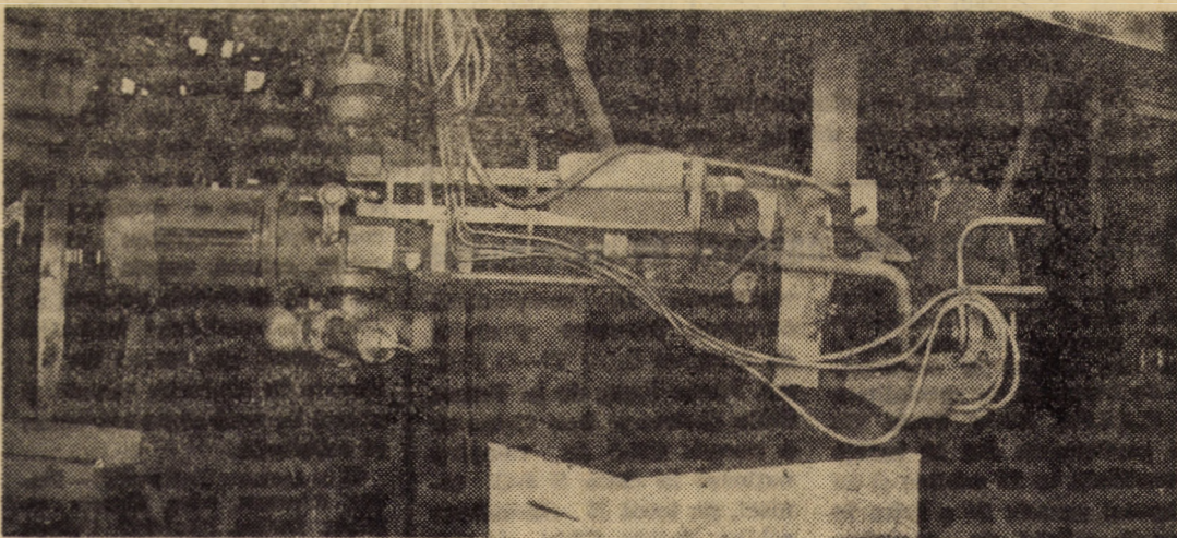
În imagine una din instalațiile de preparare a amestecurilor autointăritoare, pe bază de rășini furanice, folosite în secția turnătorie a Fabricii de utilaj metalurgic și turnătorii Sibiu
