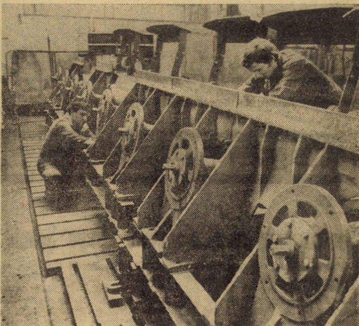
Întreprinderea „Independența” Sibiu. În fotografie, în faza de montaj, unul din utilajele de mare complexitate pentru industria metalurgică, destinat exportului. Foto: Fred NUSS
