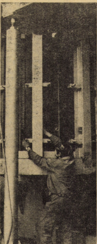
Secvență de muncă din secția utilaj metalurgic, a întreprinderii „Independența” Sibiu: Se efectuează ultimele verificări la modelul pentru granulatorul concasor de Ø 1 250 mm, destinat exportului Foto: Fred NUSS
