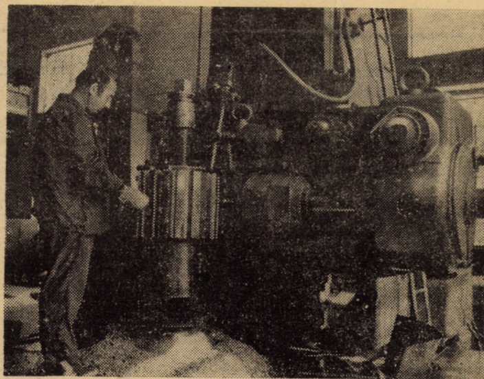
La o mașină de frezat piese de mari dimensiuni, din secția mecanică II a întreprinderii „Independența” Sibiu, frezorul Ioan Moldovan, muncitor cu îndelungată experiență profesională, execută roți dințate la un înalt nivel calitativ, componente ale unor utilaje destinate exportului
