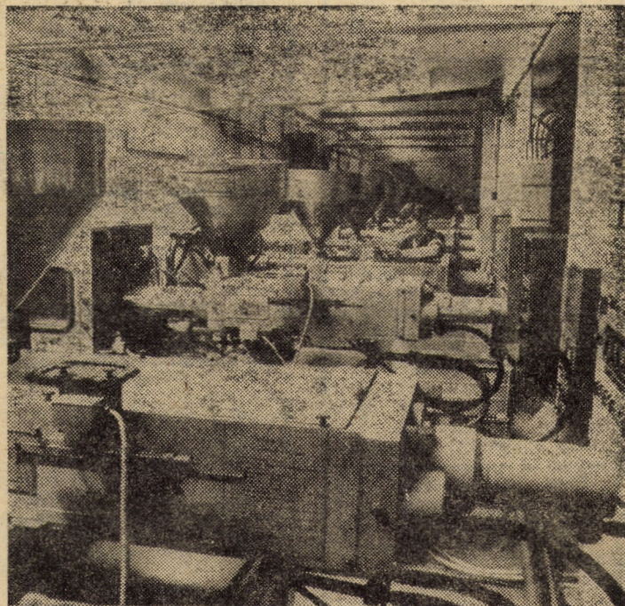
Linie modernă cu mașini de injectat mase plastice din compartimentul articole de scris de la „Flaro” Sibiu
