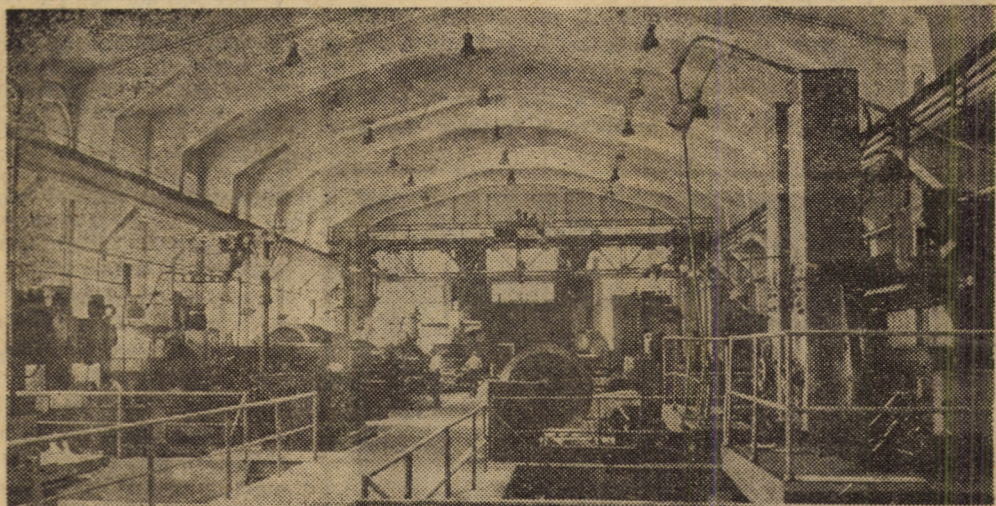
Vă prezentăm o imagine din sectorul utilaj greu, atelierul de prelucrări prin așchiere, al întreprinderii „Independența” Sibiu
