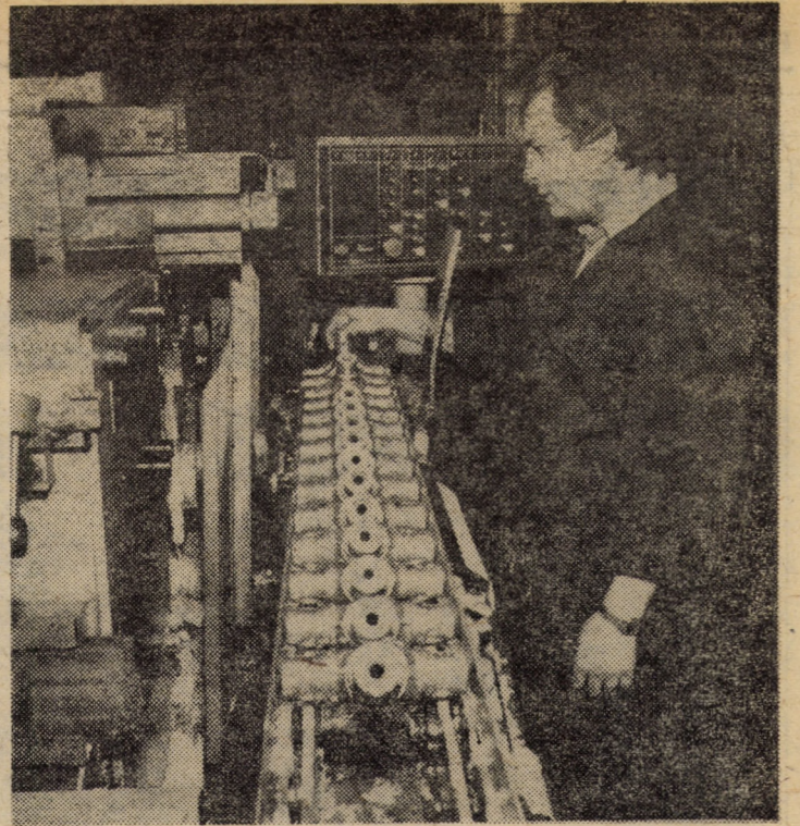
I.P.A. Sibiu - locul de muncă unde se prelucurează cu o mare precizie crucele cardanice, reper important în ansamblul organelor de transmisii ale autovehiculelor Foto: Fred NUSS
