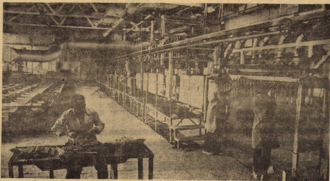
Vă prezentăm o imagine de ansamblu a liniei de cromare dură pentru tije amortizoare telescopice de la I.P.A. Sibiu
