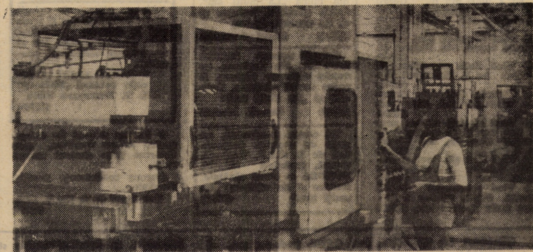
Întreprinderea „Independența” Sibiu, secția lanț cu role. Operațiunea simultană de decupare și perforare a ecliselor pentru lanțurile cu role se realizează cu ajutorul unei prese, produsă de întreprinderea mecanică Sibiu
