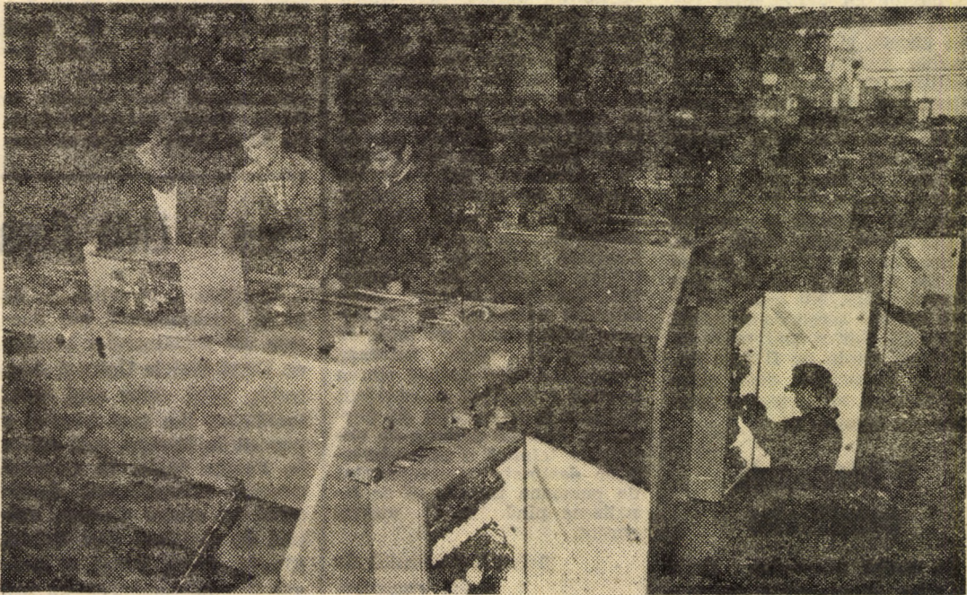
Întreprinderea „Mecanica” Sibiu. Un nou lot de foarfeci ghilotină tip FG 825, aflate în fază de montaj general și finisaj, produse destinate exportului Foto: Fred NUSS
