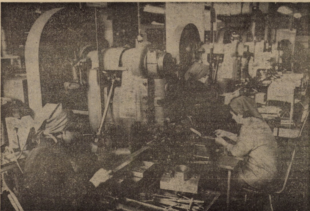
Vă prezentăm linia de imprimat și perforat ace — operație de înaltă precizie, efectuată în cadrul atelierului ace cusut pentru mașini, secția metal II a întreprinderii „Flamura Roșie” Sibiu Foto: Fred NUSS
