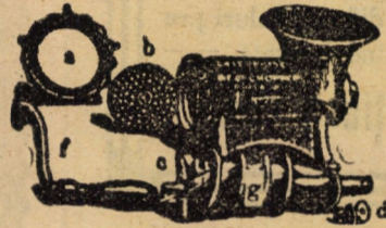
Partile constitutive dela mașina de tocat carne. a) Inel de capac, b) Disc găurit, c) Cuțit, d) Ș rof dela întorcător, e) Întorcător, f) Melciul, g) Tăp. — Fiecare să capătă separat. —
