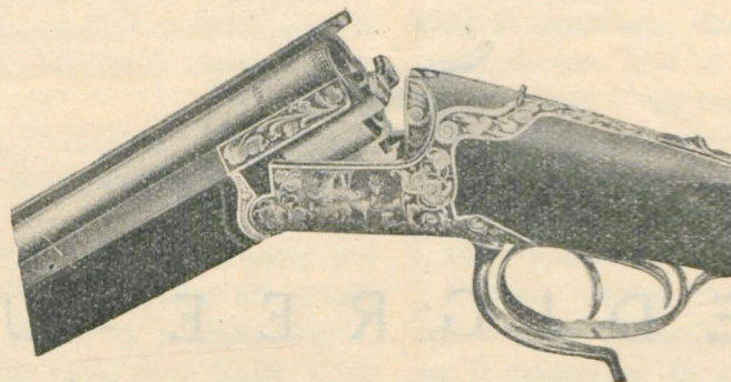
Inchișător cu dublu zăvor.
