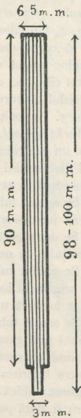
Fig. 3 Bolț de oțel
