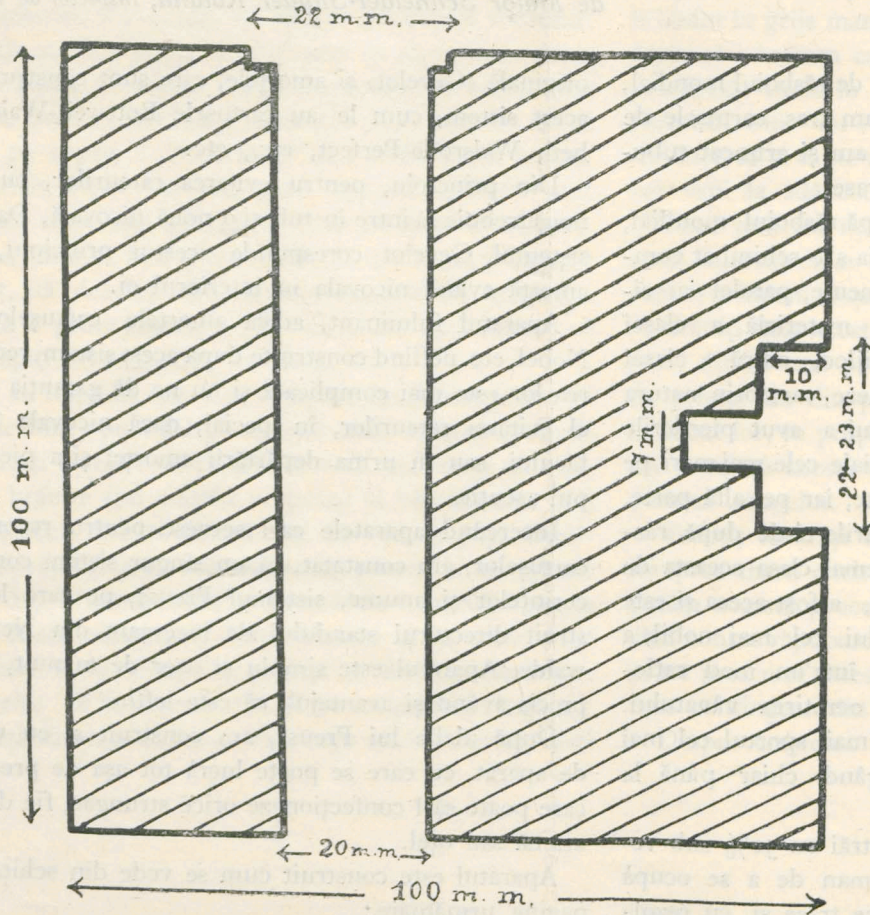
Fig. 1 Bloc din lemn de frasin 100 × 100 × 100 m. m.
