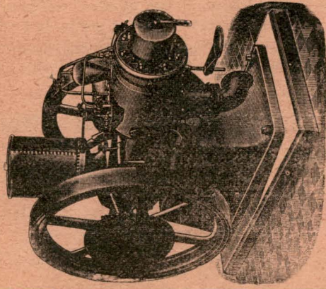
Patent „Corona“ motor.
