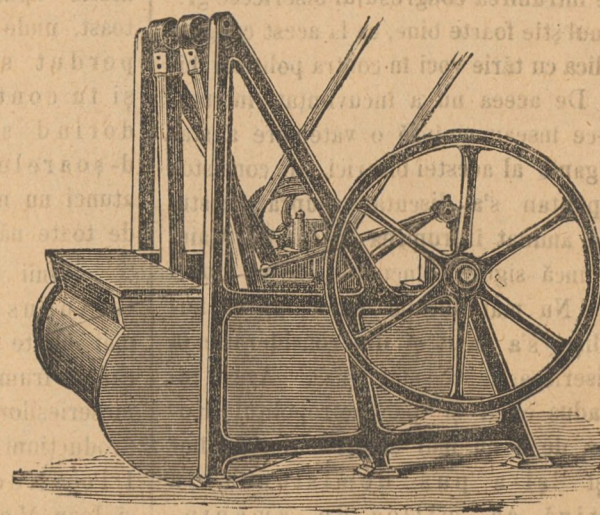
Piuă universală.
