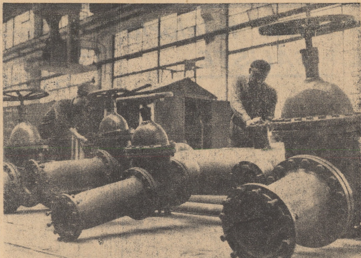
Secția construcții metalice a Uzinei mecanice Gaz metan — Mediaș. Se lucrează la montarea colectoarelor pen-tru stațiile de reglare gaze, destinate rafinăriilor de petrol.
