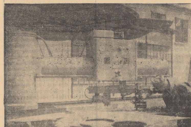
Mașină de debitat flanșe — invenția Szumilas
