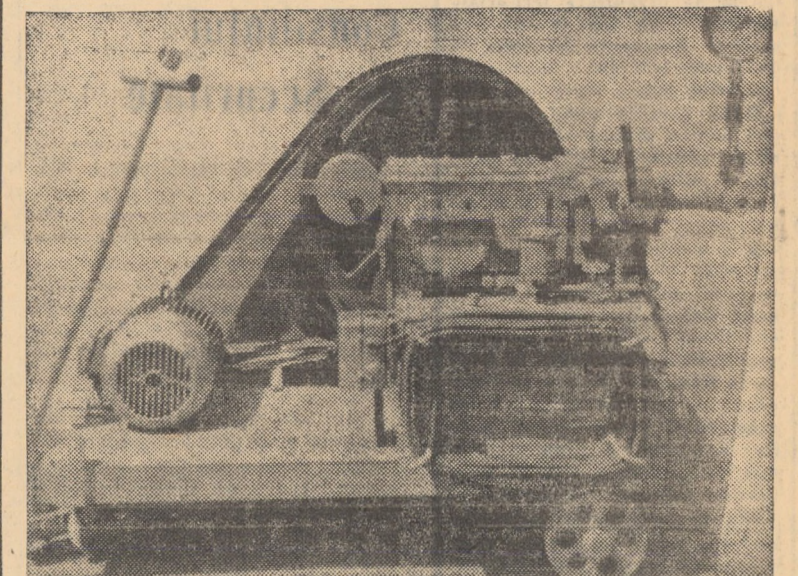
Pompă de 1000 atmosfere.
