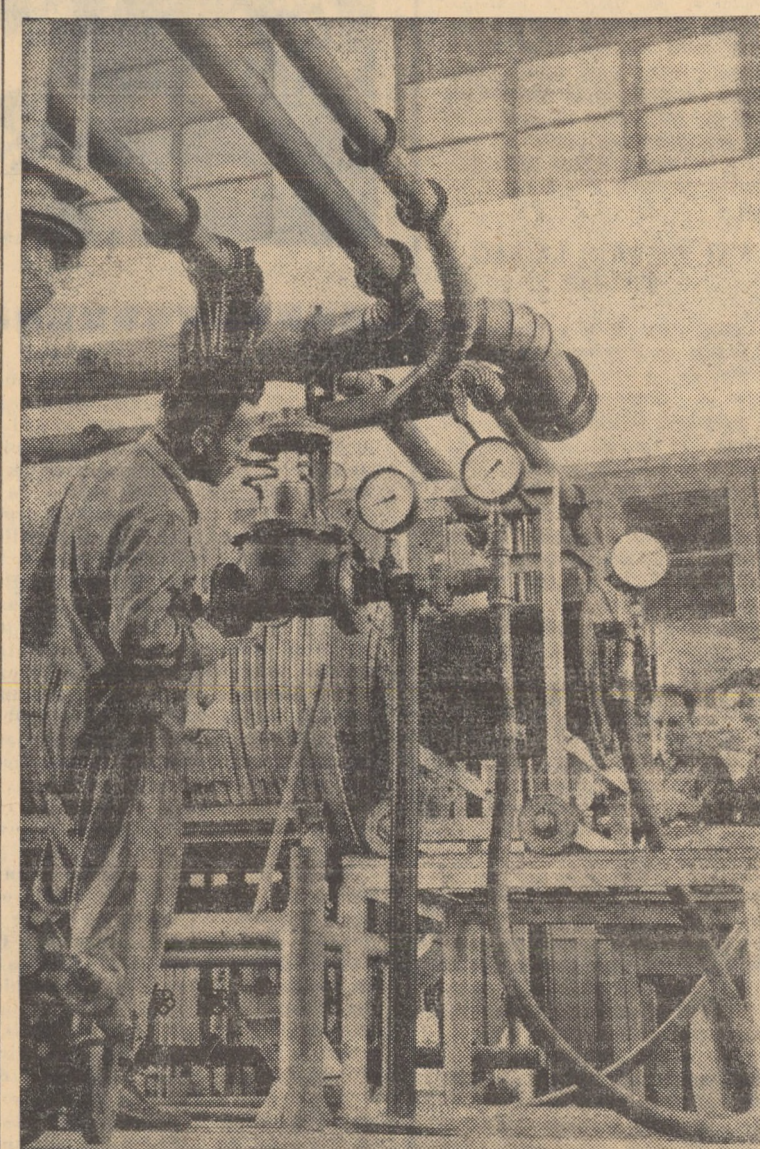
Laboratorul termotehnic al Uzinei mecanice gaz metan — Mediaș. Aici se fac încercări și măsurători la arzătoare, reguletoare pentru gaz metan.
