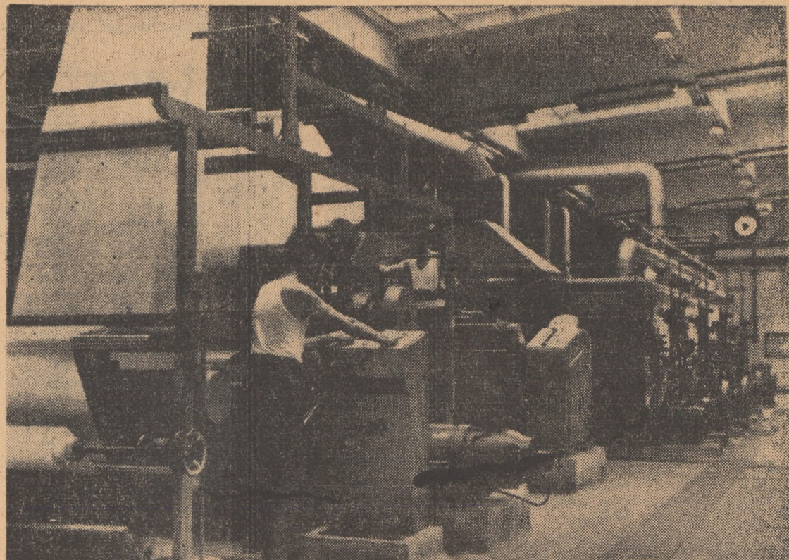
Peste 10.000 mîl țesături de mătase trec în 8 ore prin această mașină de uscat la întreprinderea „Mătasea roșie” din Cisnădie
