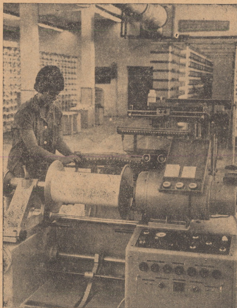
Intr-una din noile hale construite la unitatea a II-a de la fabrica „Drapelul roșu” Sibiu au fost montate mașini de urzit sectionale. Spre deosebire de utilajele mai vechi, noile mașini realizează urzeala pe o bobină care apoi este introdusă direct în mașina de tricotare, eliminîndu-se în felul acesta o fază de lucru intermediară
