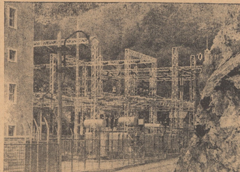
Fantezia vegetală a pădurii trece firesc în dantelăria ingenioasă a liniilor de curent care pleacă de la hidrocentrala Sadu V Foto: GEORGE STOICESCU
