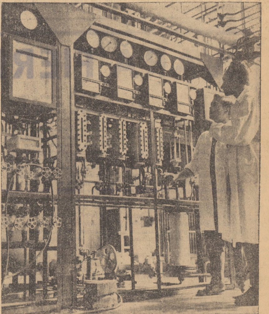
Instalația pentru sîndul valorificării acetonitrilului din secția „sinteze organice” a Institutului „Chimigaz” din Medias
