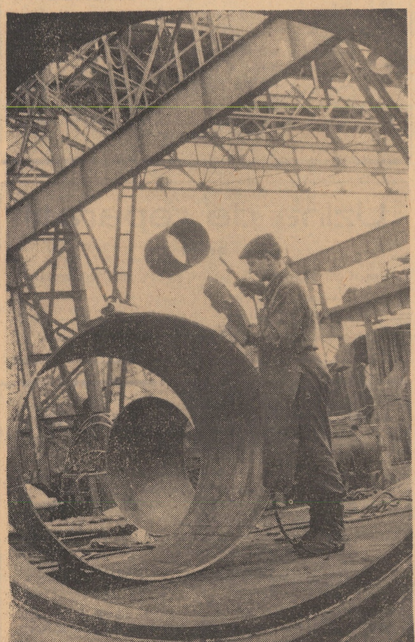
Lucrări de asamblare a virolelor la cazangeria uzinei „Indepednța” Sibiu
