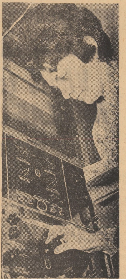
Cu ajutorul unei aparaturi speciale, în laborator pentru determinarea parametrilor emailurilor sînt efectuate analize termo-diferențiale, urmărindu-se punctele de transformare, procese exoterme și endoterme în timpul încălzirii diverselor materiale
