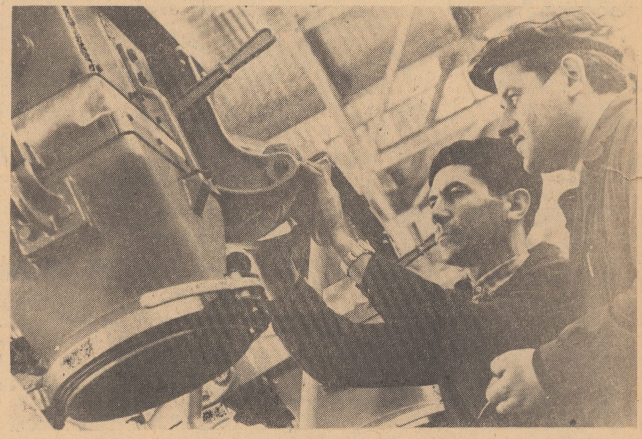
În gama variată a producției de bascule, produse de uzina „Balanța” din Sibiu, se include și balanța semi-automată de înscuit de 100 kg, mult apreciată și peste hotare. În fotografie: produsele în faza montaj
