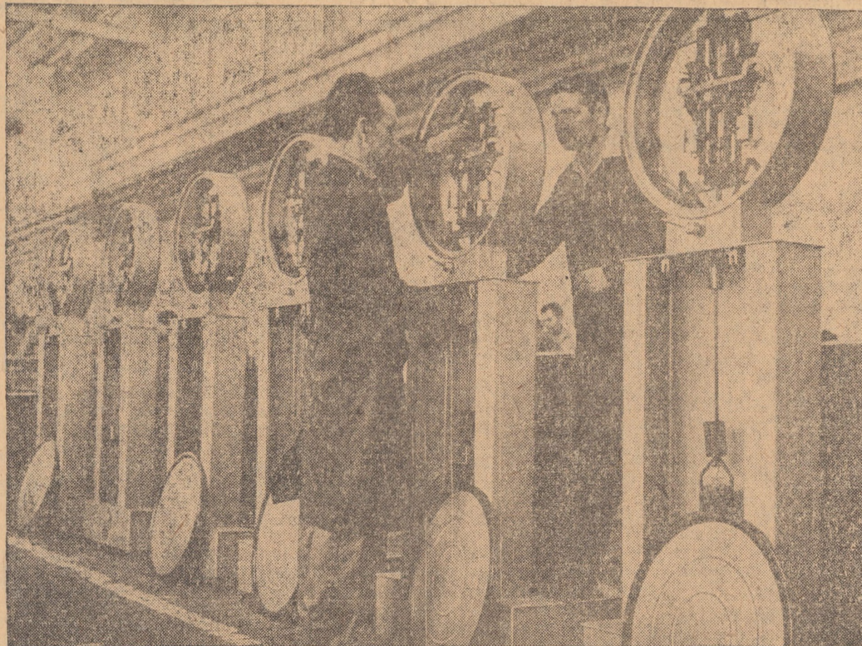
Montajul și ajustarea unui lot de bascule semiautomate la uzina „Balanta” din Sibiu
