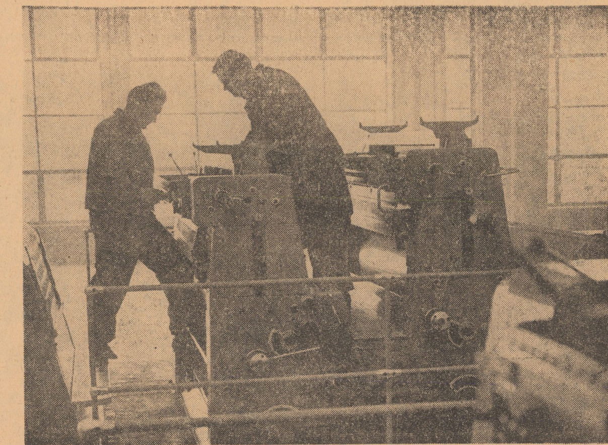
Montarea noilor utilaje — mașini ofset cu imprimare în două culori — la noul sediu al întreprinderii poligrafice Sibiu de pe șoseaua Albi Julia
