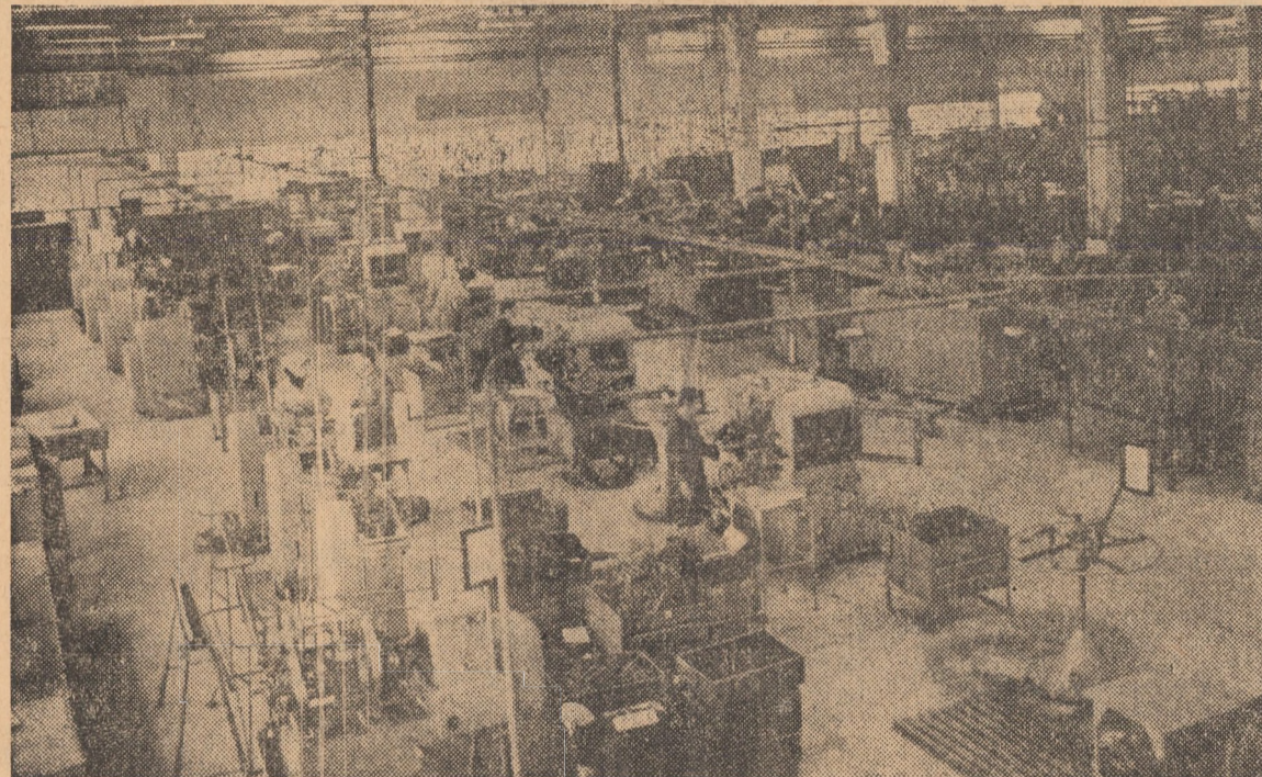
Uzina de piese auto. Aspect din secția de furnici înfășurate la rece, secție nou intrată în funcțiune
