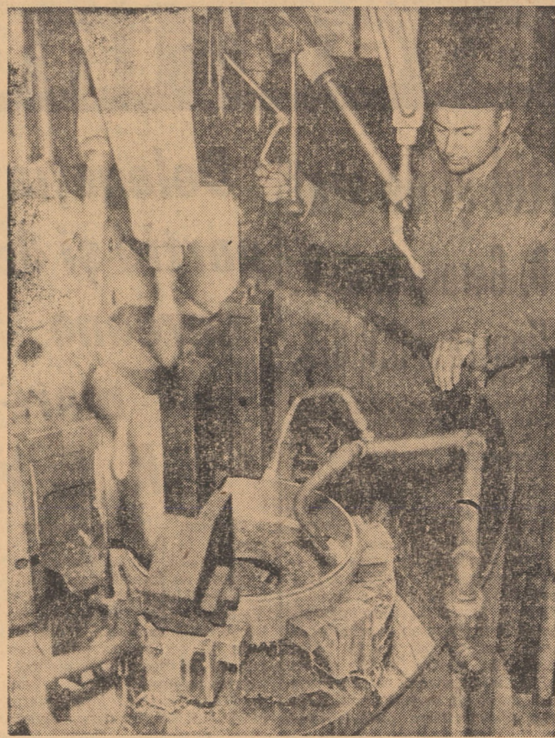
Uzina mecanică Mirșa. Strungirea tamburilor de frână folosii la mare productivitate, care pot realiza cca. 300 piese într-o zi. Foto: HORST BUCHFELNER
