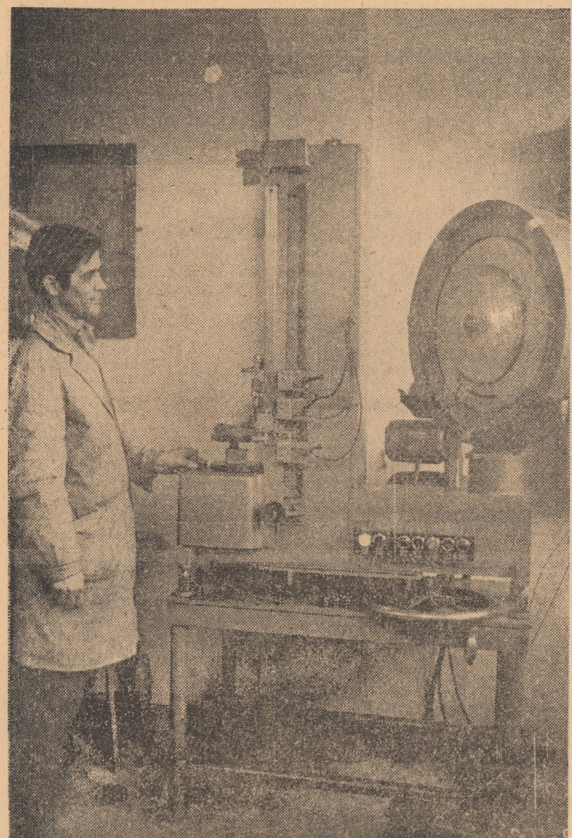
Uzina de piese auto Sibiu este înzestrată cu aparate și utilaje moderne. În clișeu aparatul mecanizat de controlat arcuri după diagramă și săgeată
