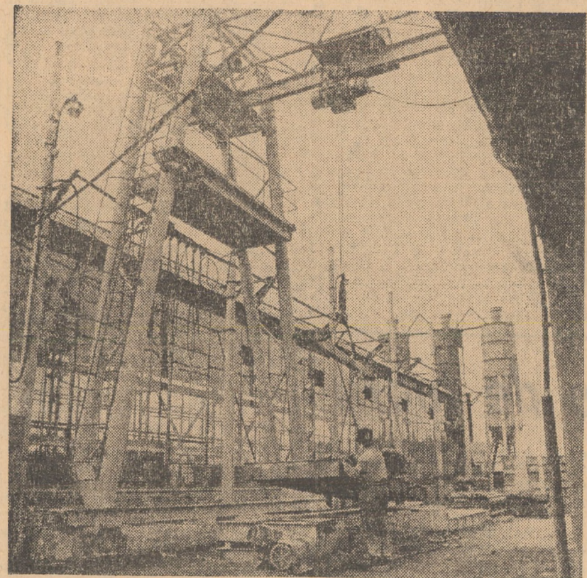
Noua hală în care se produc fiacă cu goluri din beton a întreprinderii industriale județene Sibiu, MACO unde, în anul 1971, se va realiza o producție în valoare de 14 milioane lei
