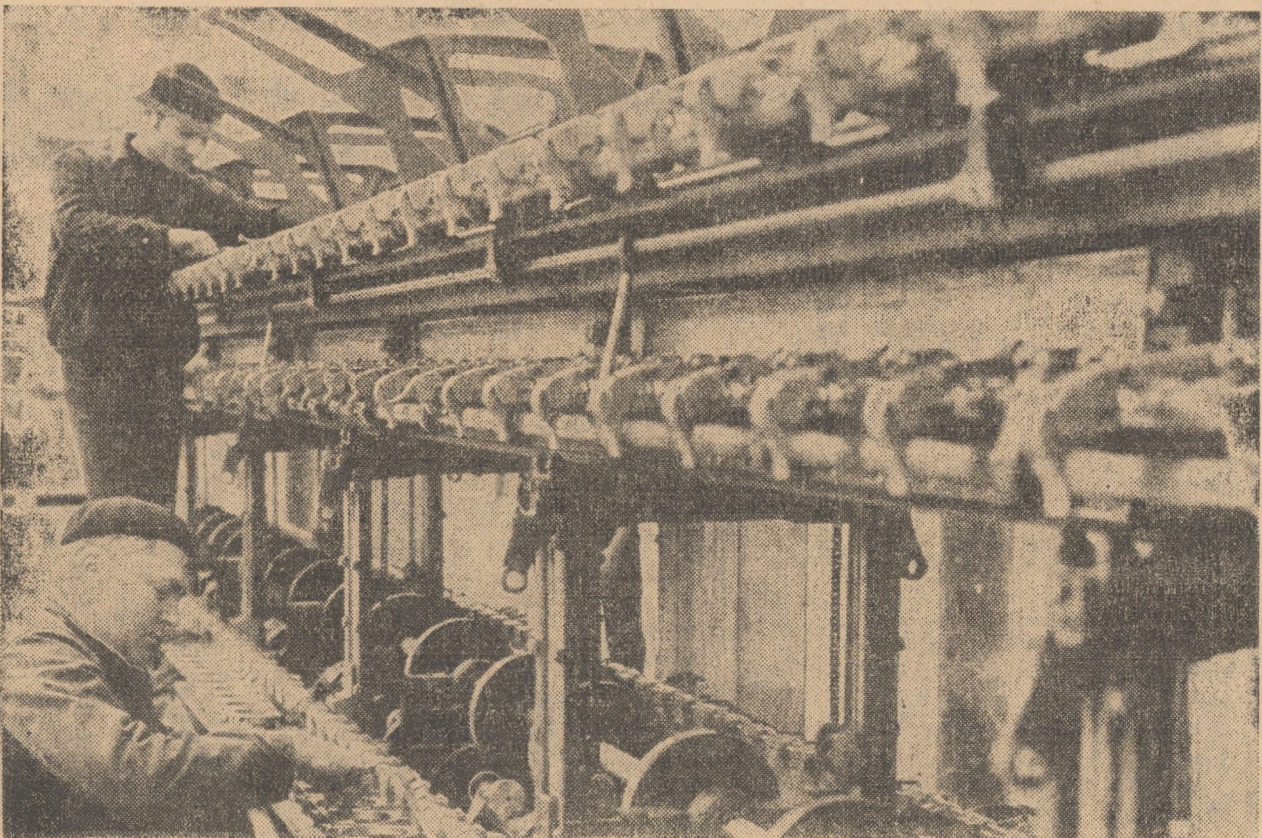
În noua hală a fabricii cardate de la Uzinele textile Cisnădie se află în curs de montare (fotografia noastră) un grup de mașini cu inele cu formate mari de bobine și viteze de debitare sporite. Noile utilaje, în parte intrate în funcțiune, vor fi incluse în ciclul de producție la sfîrșitul trimestrului II a.c.
