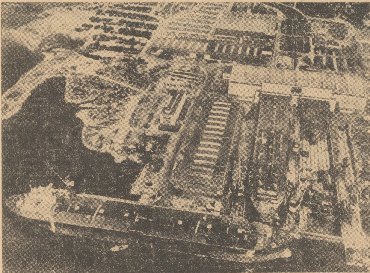
SUEDIA. La șantierele navale Arendals din Gothenburg, se construiesc în serie petoliere, toate depășind deplasamentul de 200.000 de tone. În foto: vederea aeriană a șantierei navale Arendals, cu un vas dat la apă și alte două în construcție. Un petrolier de 228.000 de tone a fost construit în 26 de săptămîni în loc de un an cum se construiesc după metodele tradiționale
