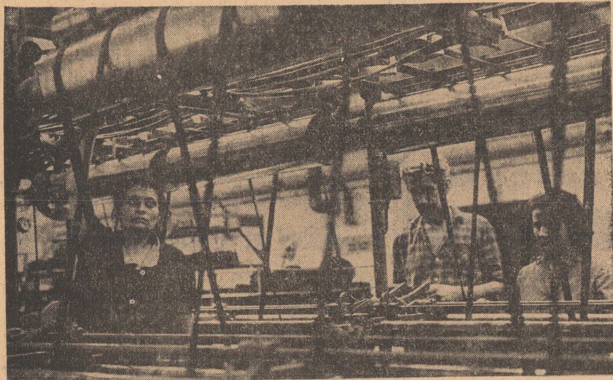
Mașina de spîlat și uscat pale din secția vopsitorie a fabricii „Libertatea” Sibiu, realizează cca 1.000 kg pale/8 ore. De aici, acestea alimentează secția filatură pieptănă
